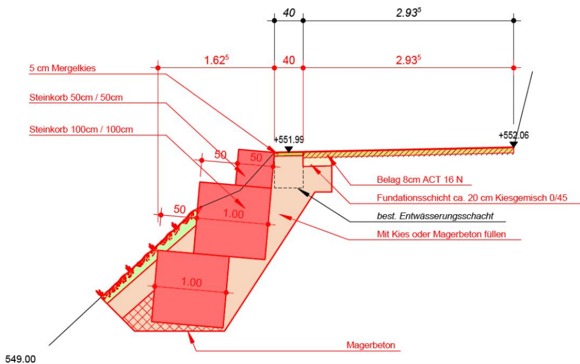
Bild 4: Massnahme Nr. 8, Querschnitt
